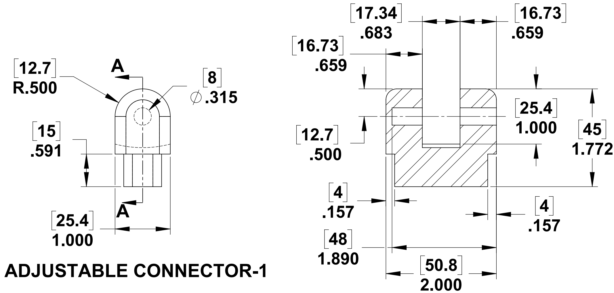
SECTION A-A
